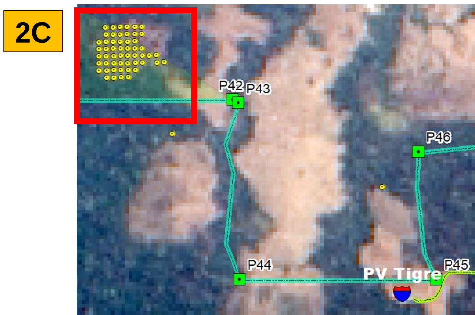
Figura 13. Mapa de Alertas de deforestación (Geobosques). Sector Qda Tigre. Agosto 2024
