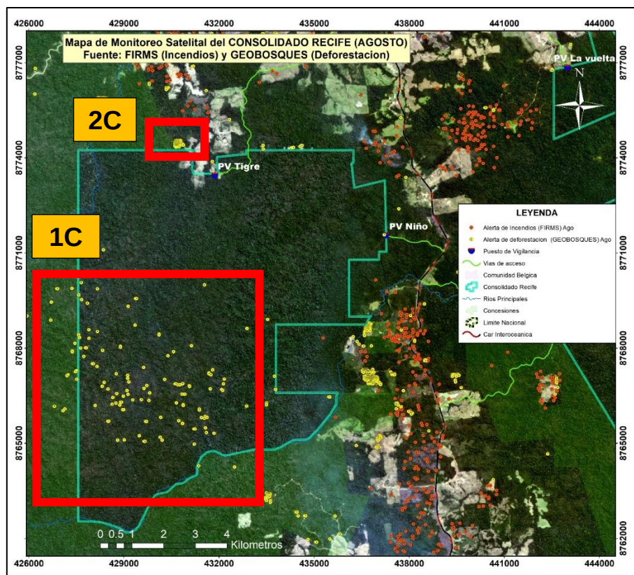
Figura 12. Mapa de Alertas de deforestación (Geobosques) e Incendios Forestales (FIRMS) En la zona Tigre-Noaya..Agosto-2024
