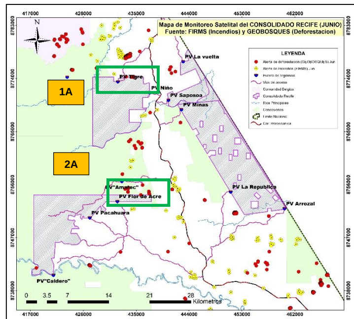
Figura 7. Mapa de Alertas de deforestación (Geobosques) e Incendios Forestales (FIRMS). Junio 2024
