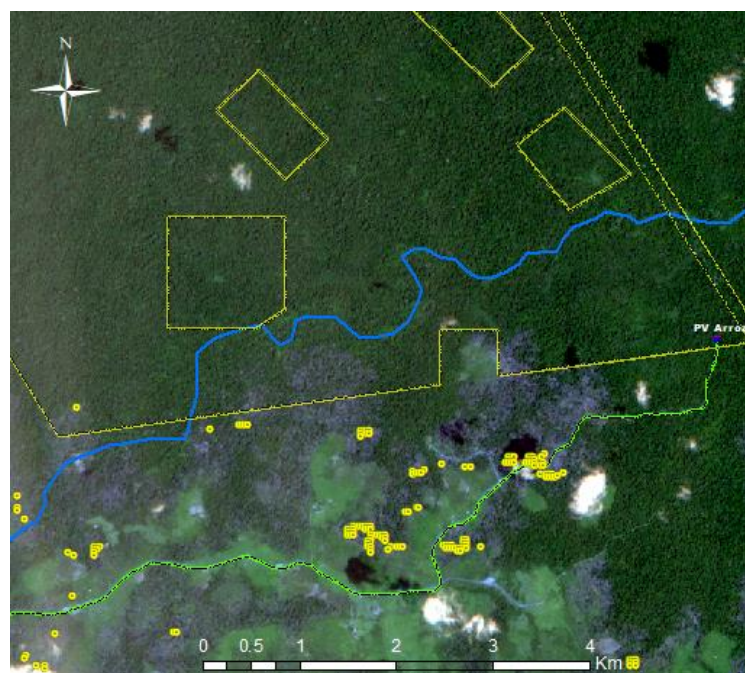
Figura 21. Imagen satelital con alertas de deforestación en el sector Arrozal. Diciembre-2024
