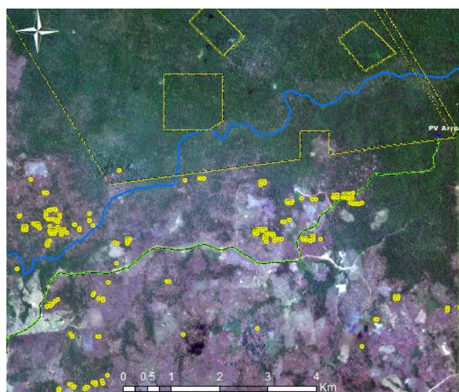
Figura 19. Imagen satelital con alertas de deforestación en el sector Arrozal. Noviembre-2024
