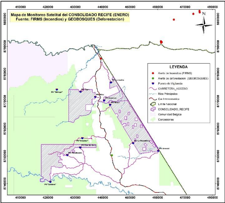
Figura 2. Mapa de Alertas de deforestación (Geobosques) e Incendios Forestales (FIRMS) Enero 2024.
