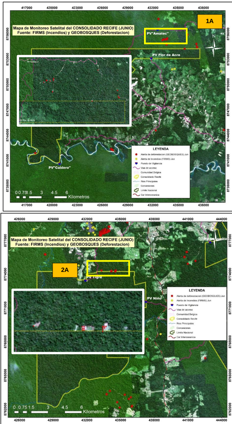
Figura 8. Mapa de Alertas de deforestación (Geobosques) e Incendios Forestales (FIRMS).
