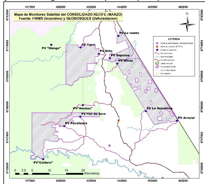
Figura 4. Mapa de Alertas de deforestación (Geobosques) e Incendios Forestales (FIRMS) Marzo 2024.
