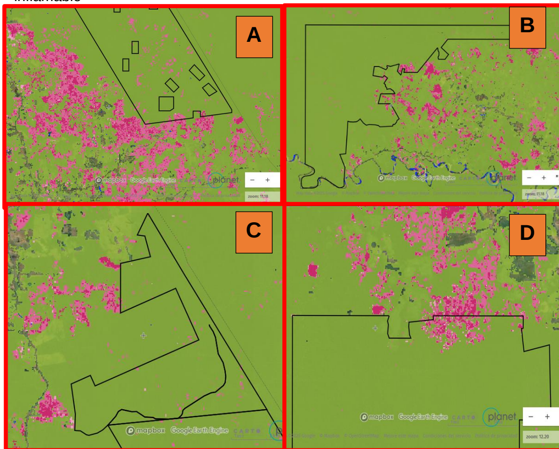
Figura 31. Alertas de Deforestación del Aplicativo Global Forest Watch en el Consolidado Recife A. Sector Arrozal-Republica B. Sector Pacahuara-Flor de Acre-Alto Alianza C. Sector Cardozo Noaya y D. Sector Tigre Noaya
