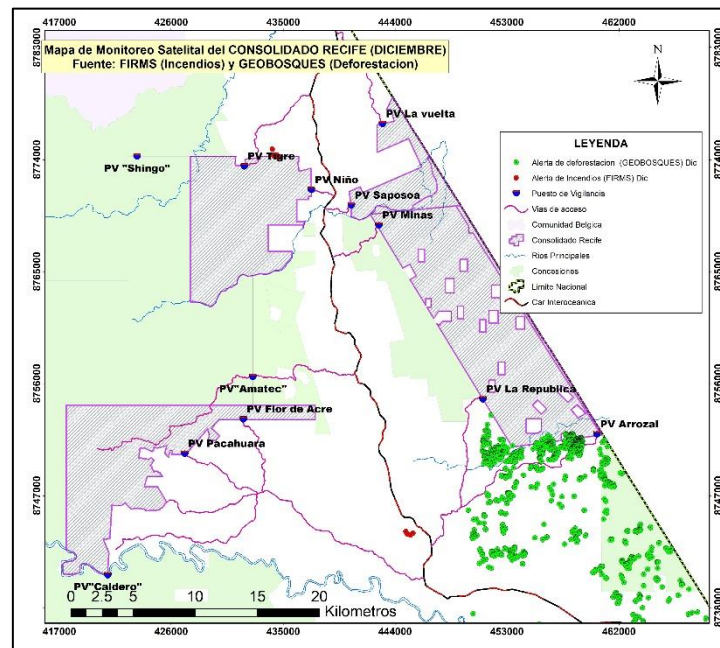
Figura 20. Mapa de Alertas de deforestación (Geobosques) e Incendios Forestales (FIRMS). Diciembre 2024
