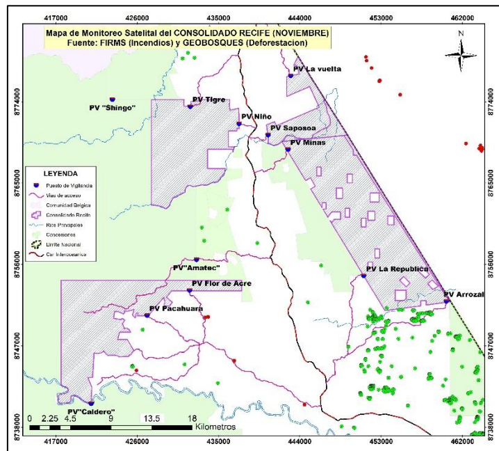
Figura 18. Mapa de Alertas de deforestación (Geobosques) e Incendios Forestales (FIRMS). Noviembre 2024
