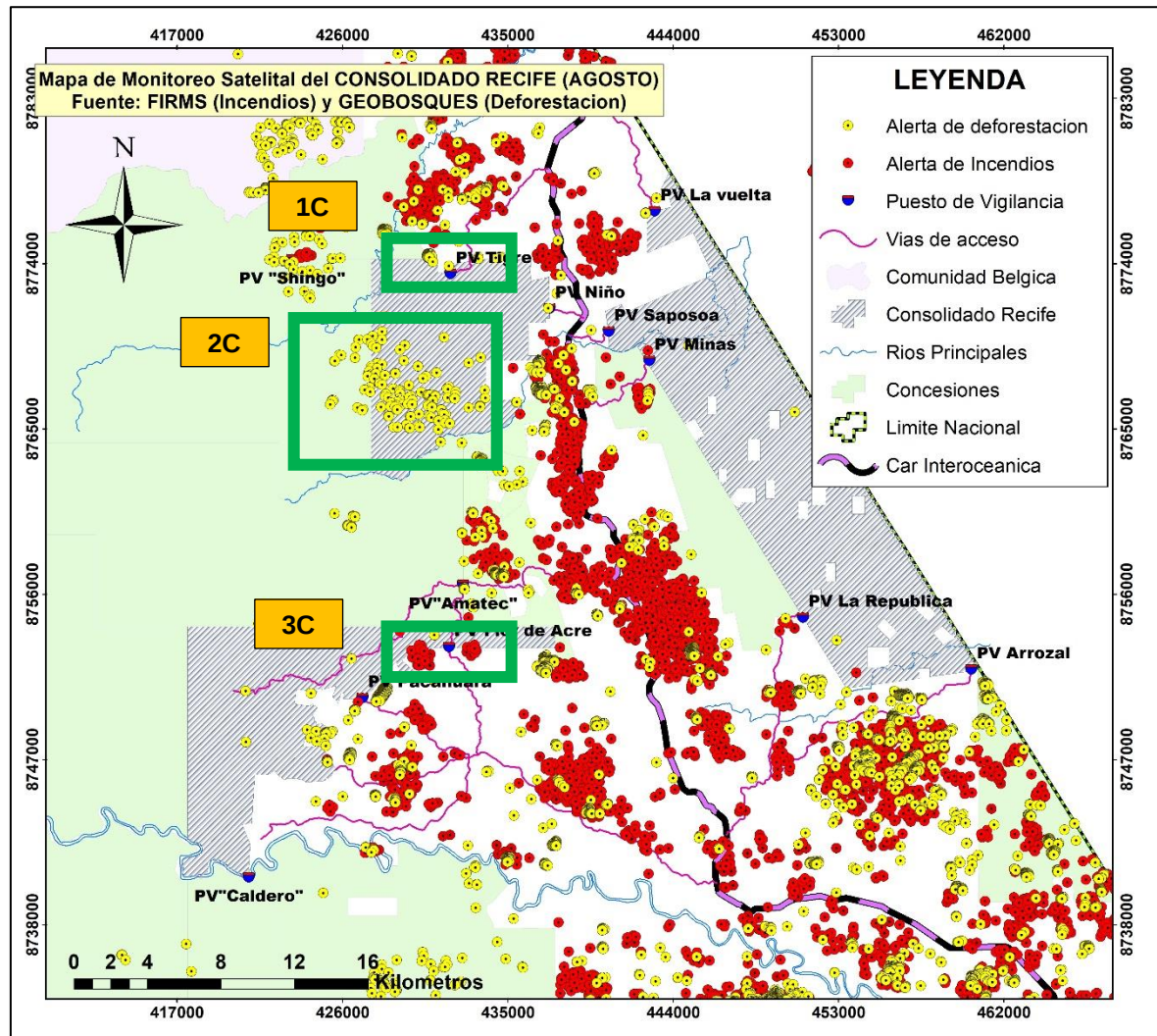
Figura 11. Mapa de Alertas de deforestación (Geobosques) e Incendios Forestales (FIRMS). Agosto 2024
