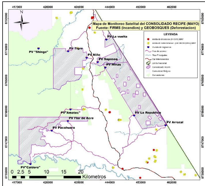
Figura 6. Mapa de Alertas de deforestación (Geobosques) e Incendios Forestales (FIRMS). Mayo 2024
