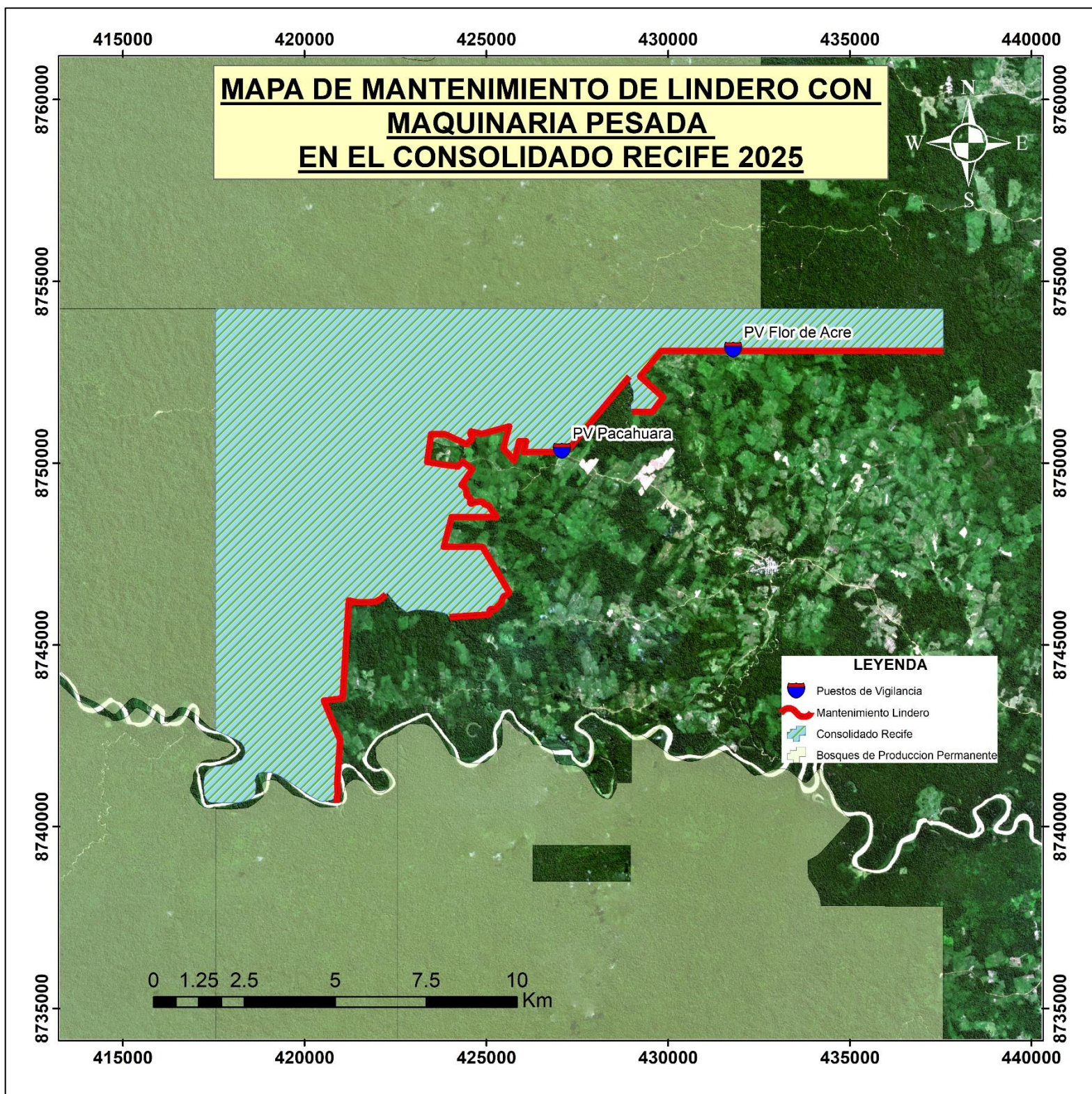
Anexo 1C: Mapa de Mantenimiento de Linderos con Maquinaria Pesada.
